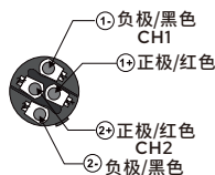
音箱螺旋插头 Speakon(NL4)
